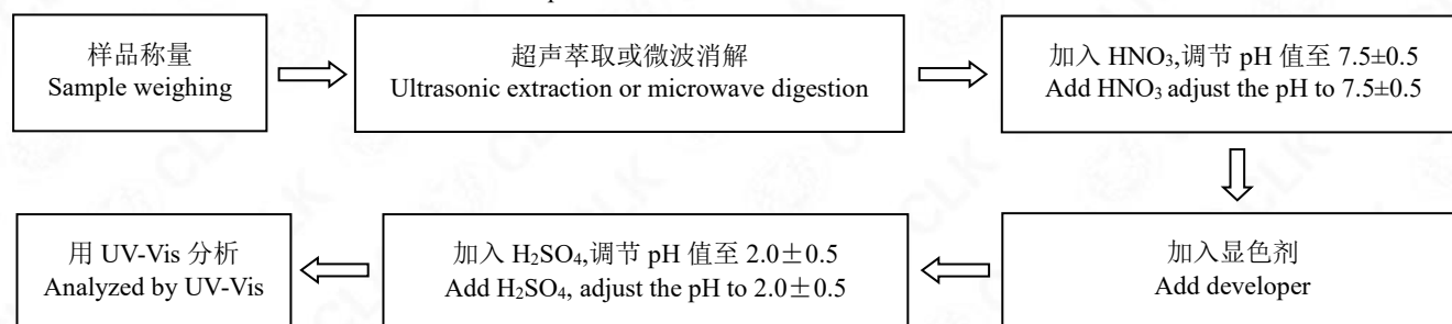
Cr 6+ 检测流程 (非金属) (Cr 6+ non-metallic test process) :
